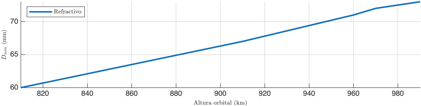
h vs D_{min} viable - Detector 2 - Configuración: 3 satélite(s), 1 telescopio(s) por satélite
